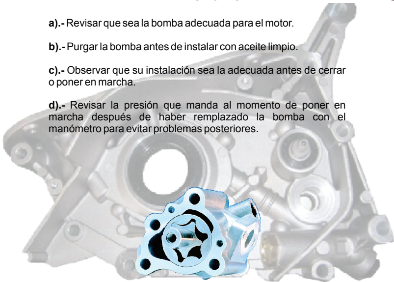
Bomba de Lóvulos
